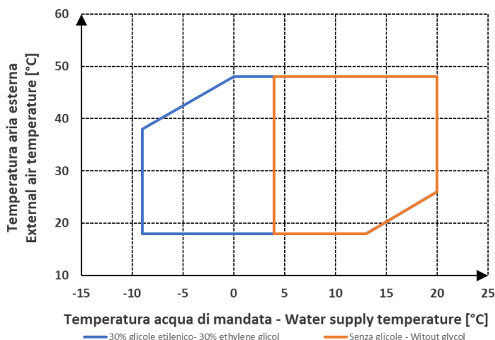
Prestazioni in freddo - Cooling performance
