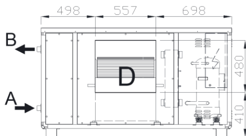
VISTA LATO MANDATA ARIA
